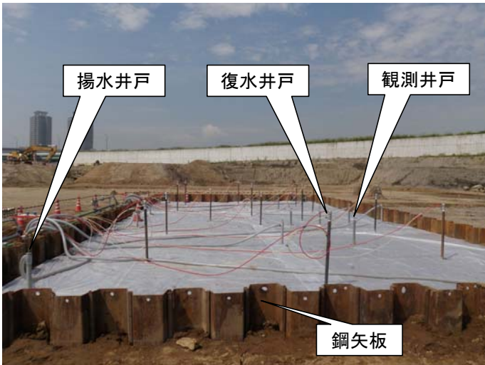
汚染地下水対策の状況
