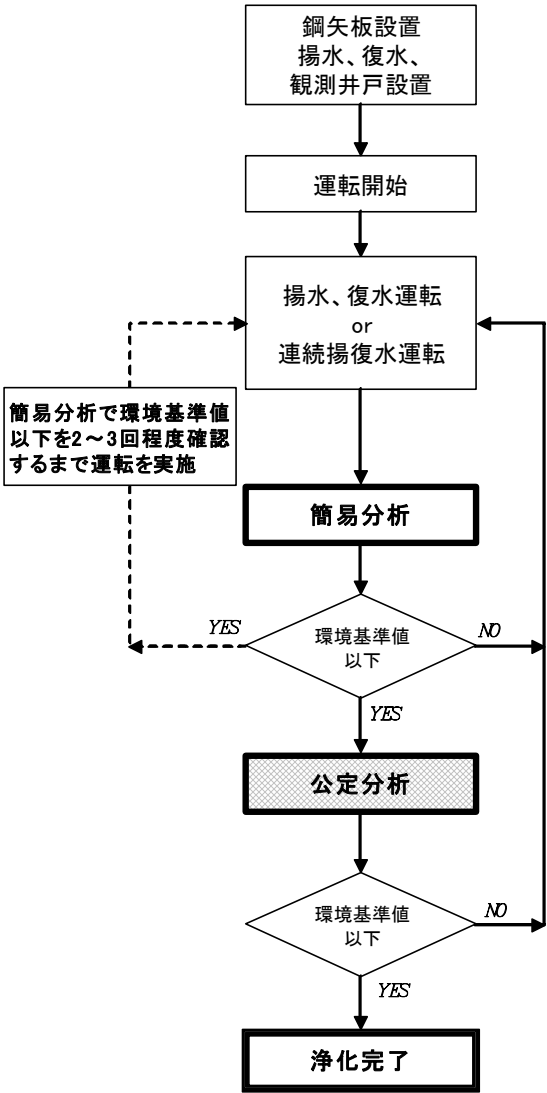
汚染地下水浄化の流れ
