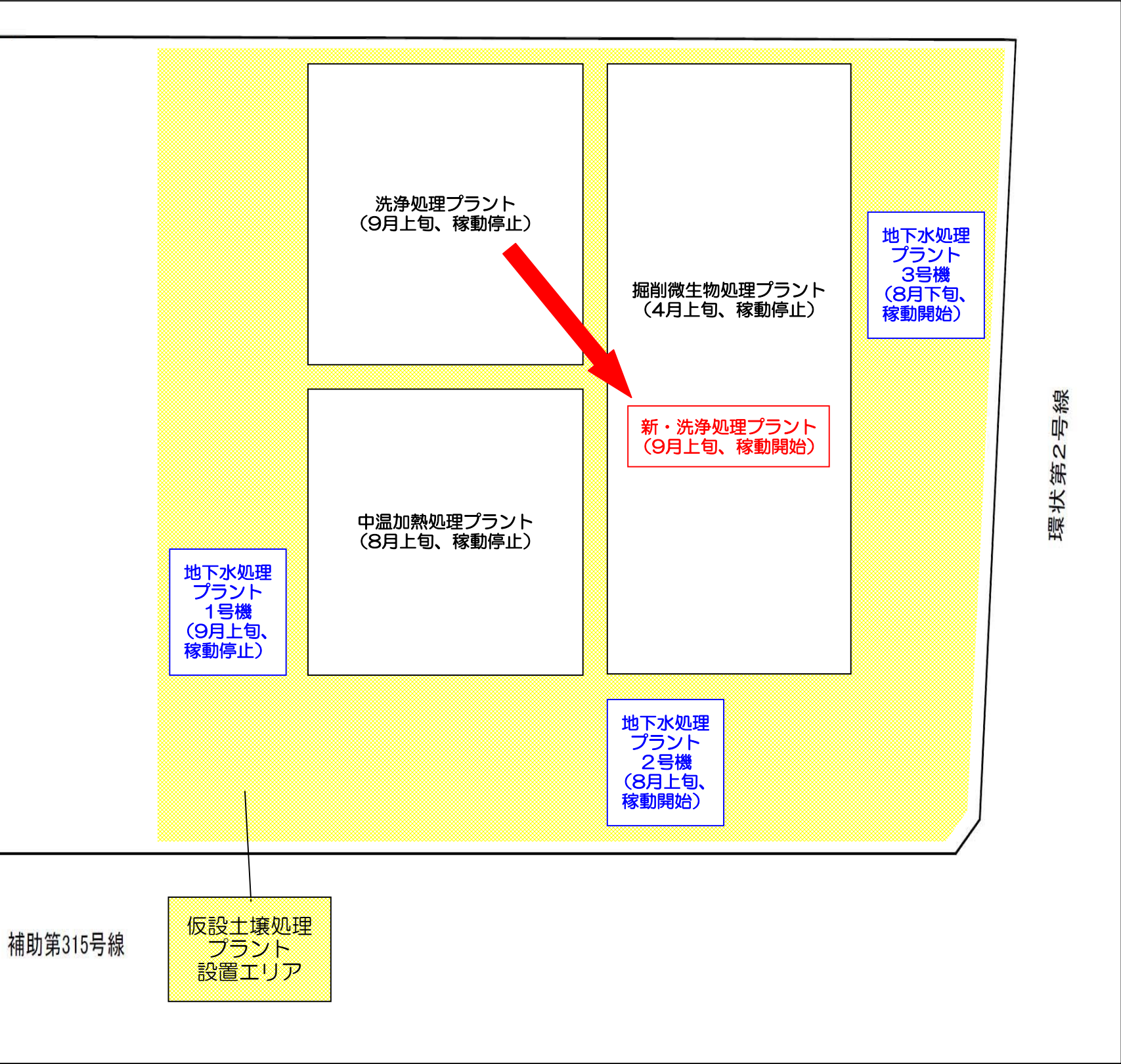
仮設土壌・地下水処理プラント概略位置図 (6街区)
