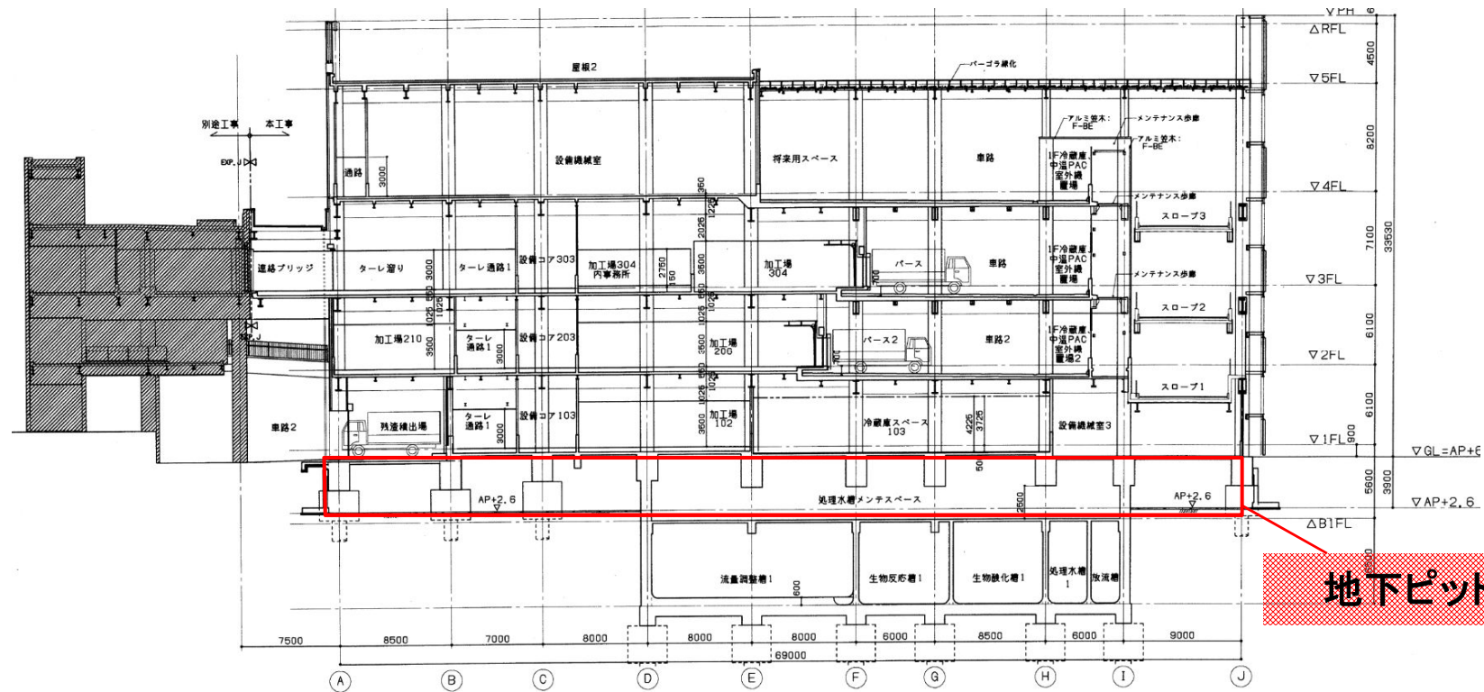
配管設置後
