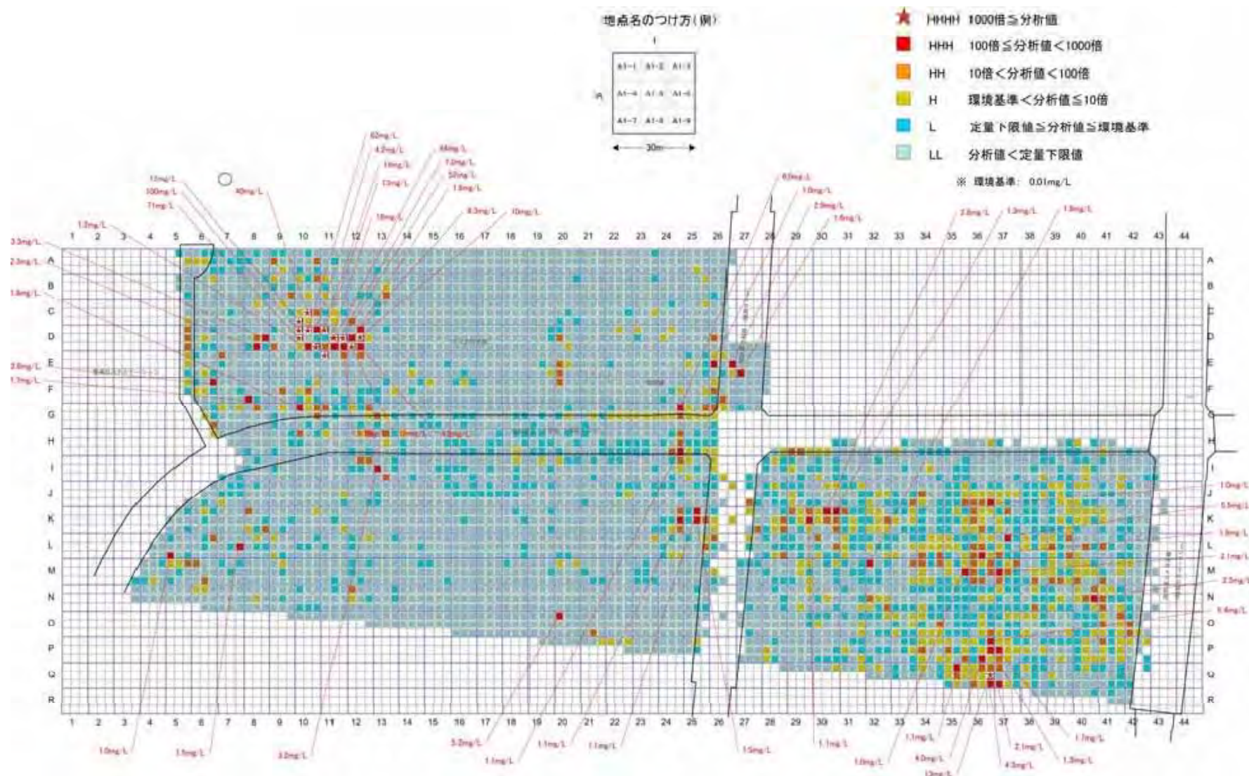
図 1 (1) 詳細調査結果 地下水 濃度分布図(ベンゼン)
