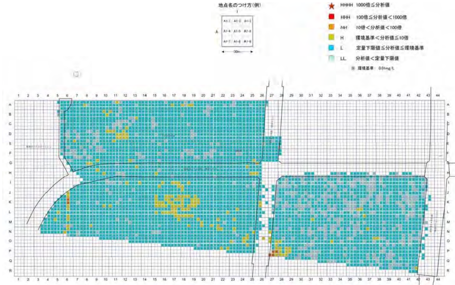
図 1 (3) 詳細調査結果 地下水 濃度分布図 (ヒ素)
