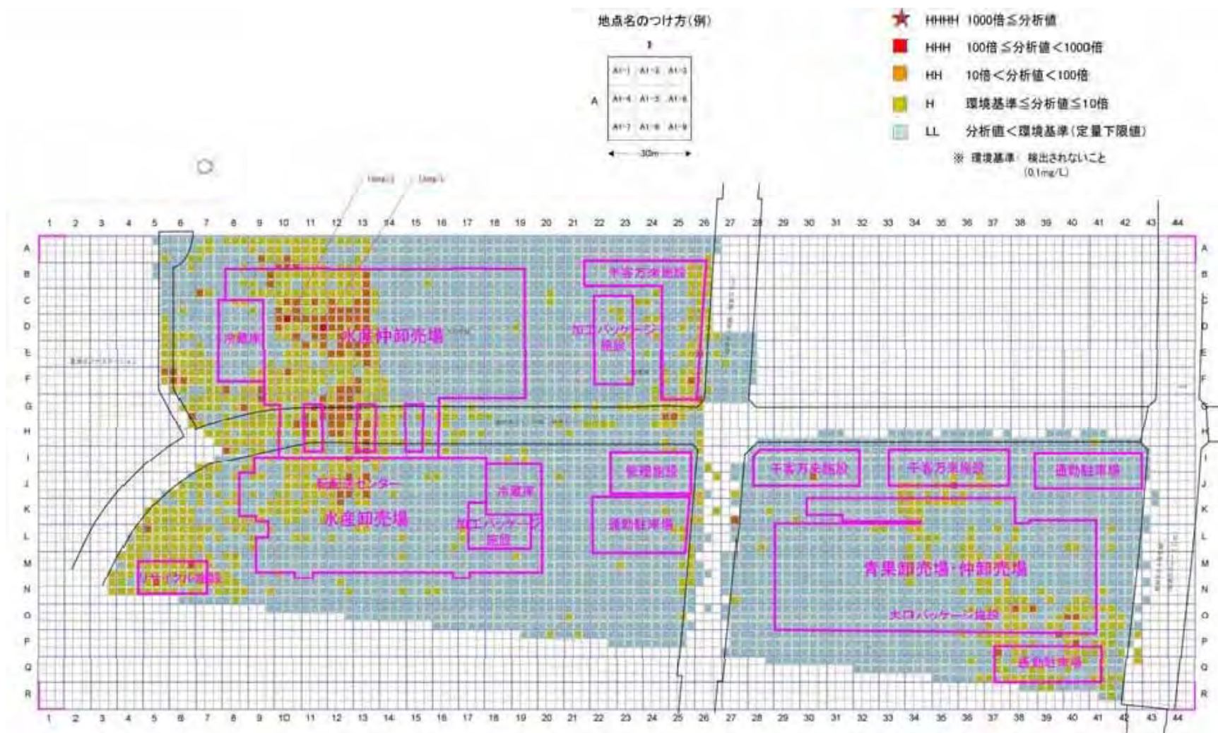
図 2 (2) 詳細調査結果 豊洲新市場施設配置と地下水濃度分布図 (シアン化合物)
