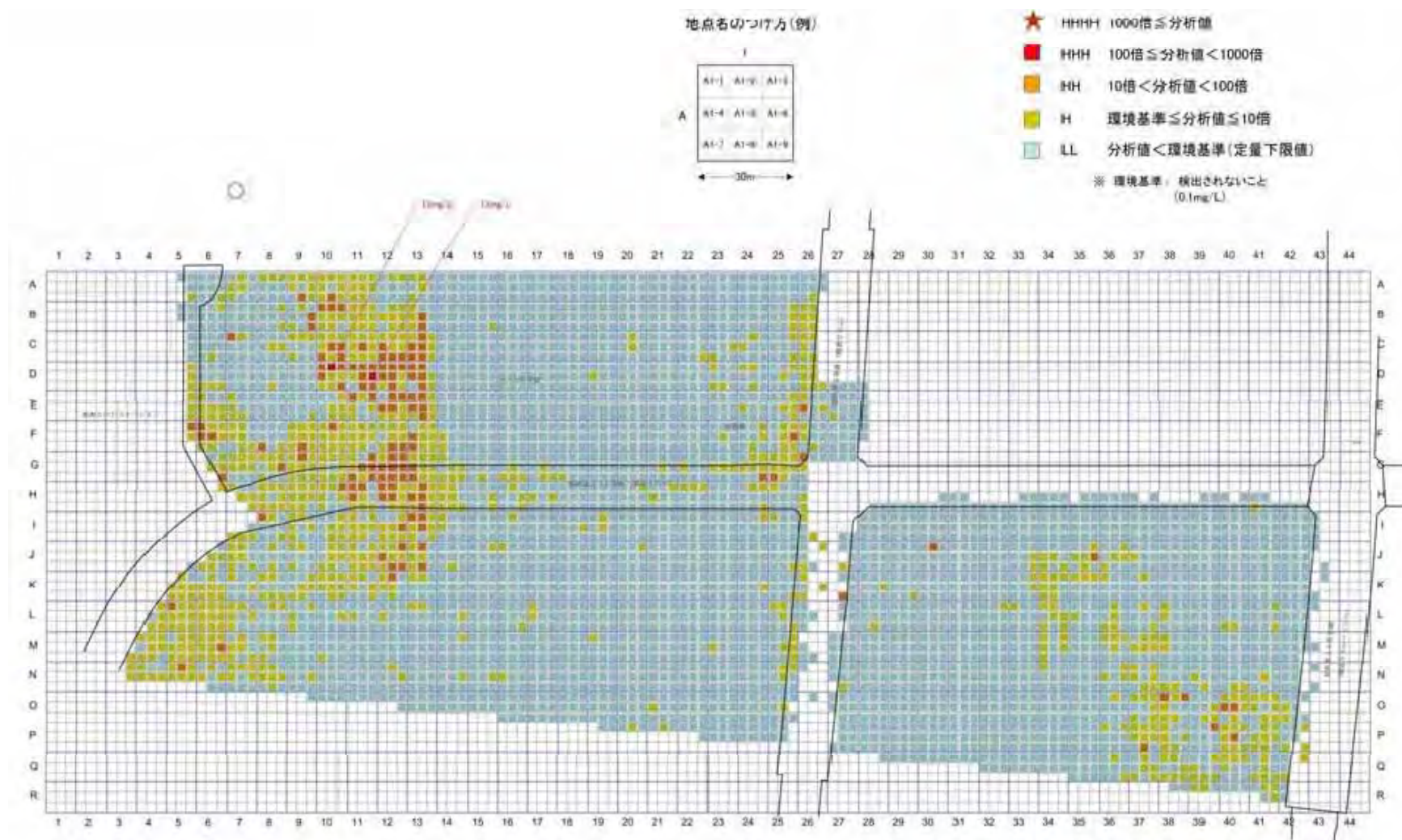
図 1 (2) 詳細調査結果 地下水 濃度分布図(シアン化合物)
