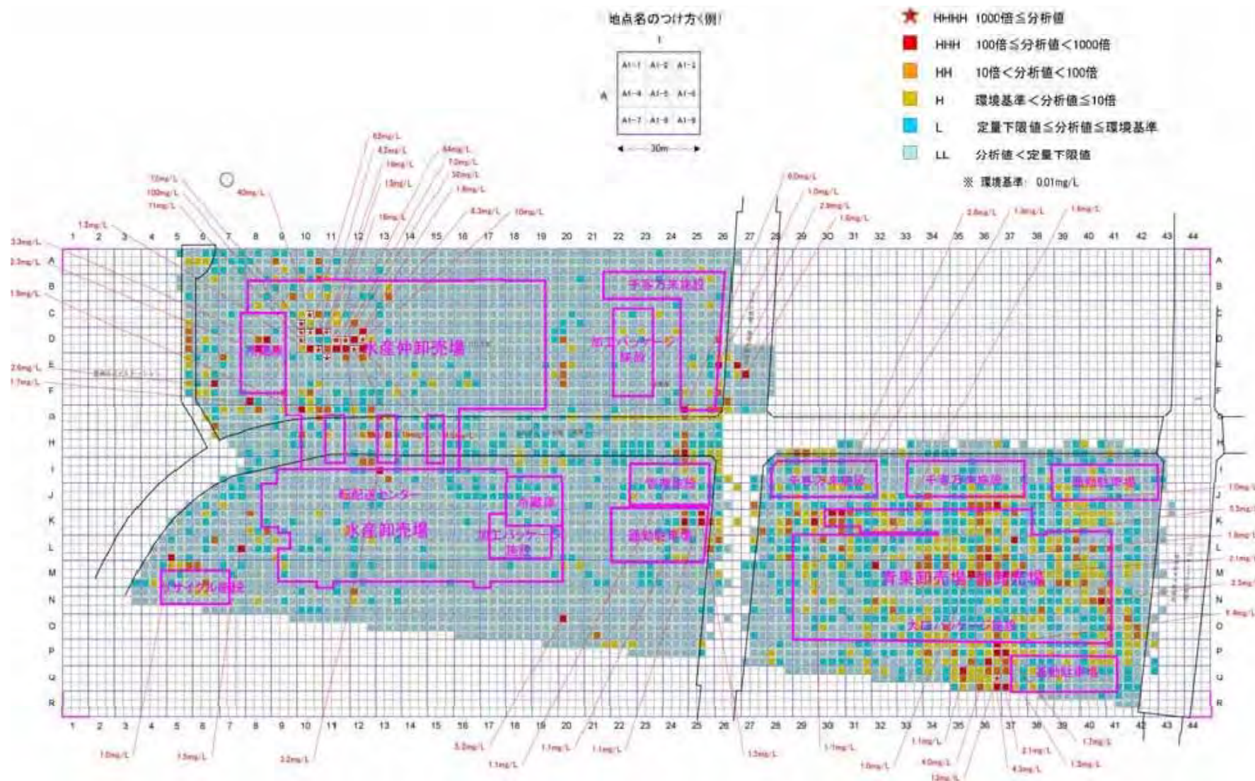
図 2 (1) 詳細調査結果 豊洲新市場施設配置と地下水濃度分布図（ベンゼン）
