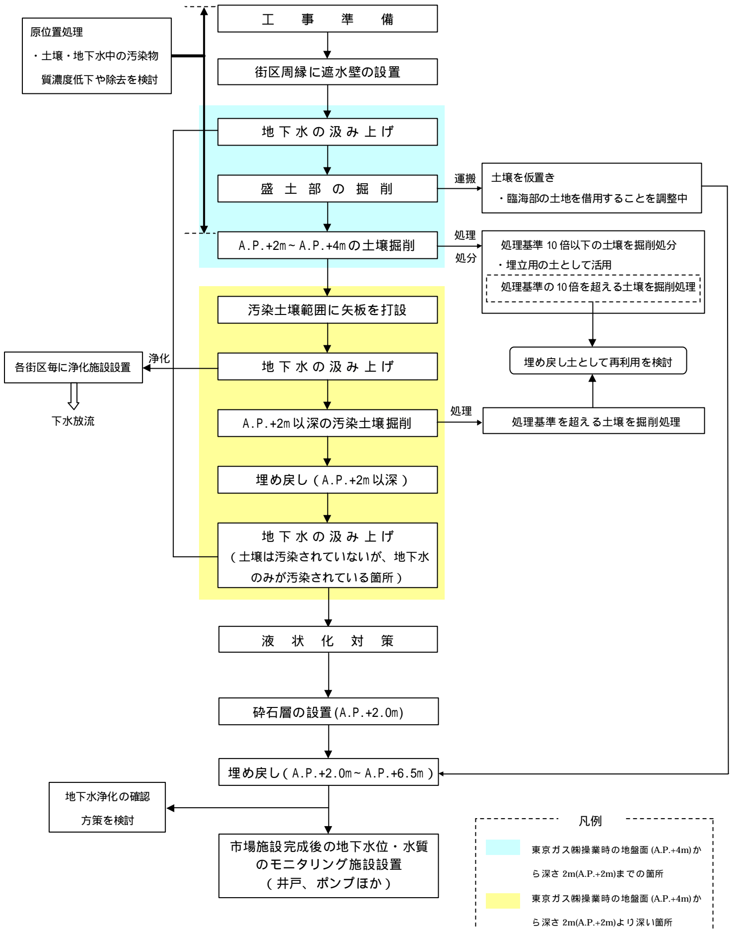
図1-1 工事の全体フロー図
