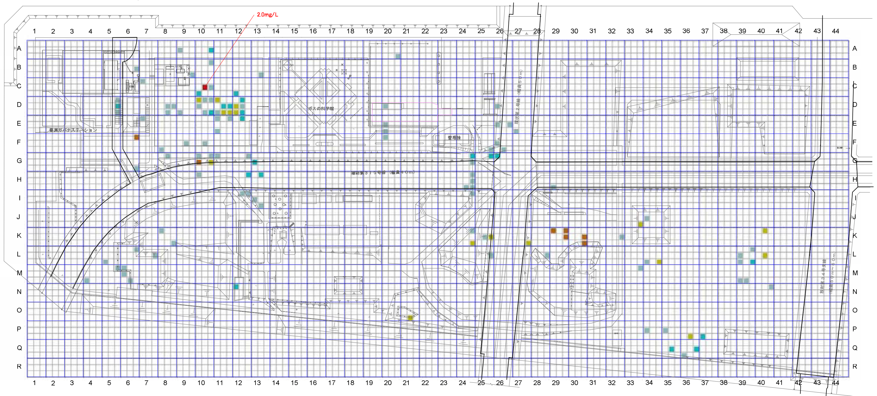
土壤溶出量 濃度分布図 (ベンゼン、工場操業時地盤面-6m)
