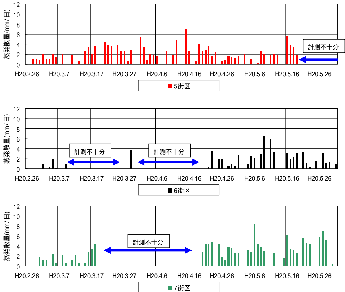
図 6.1.5 各街区における蒸発散量観測結果
