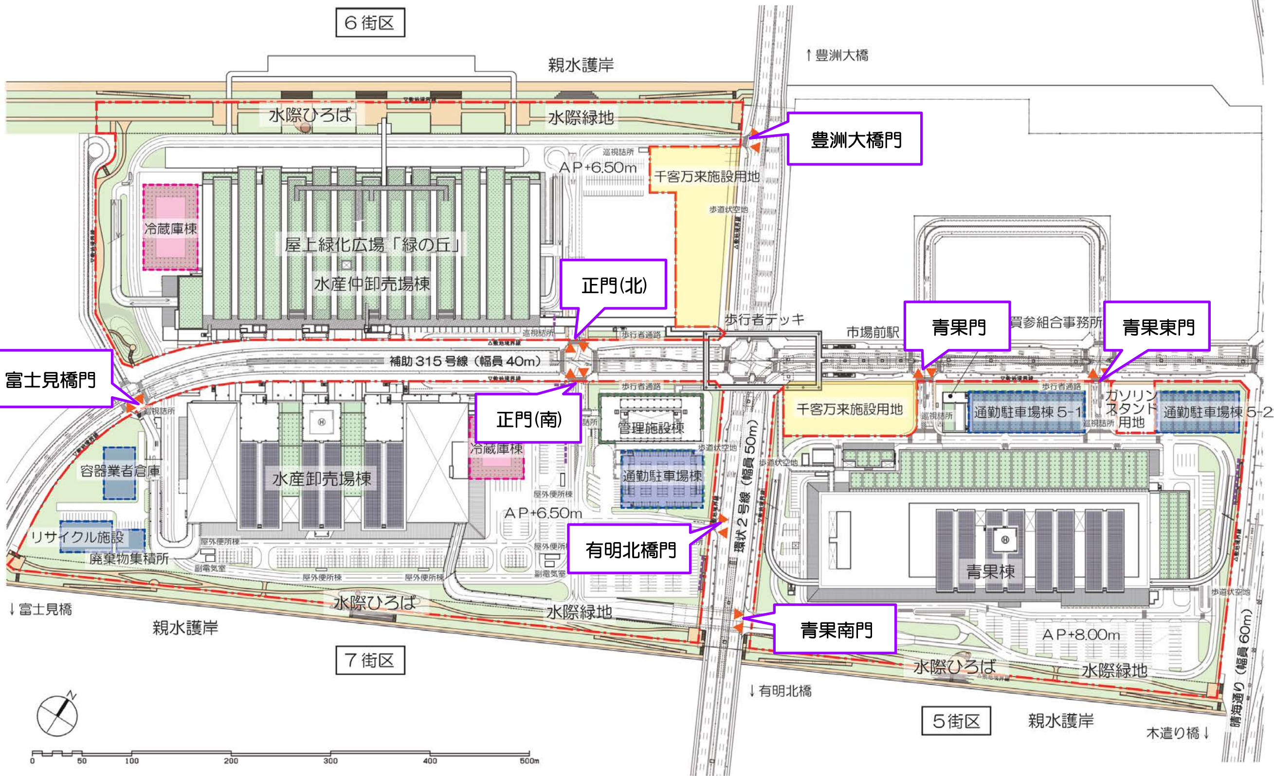
豊洲市場配置図
