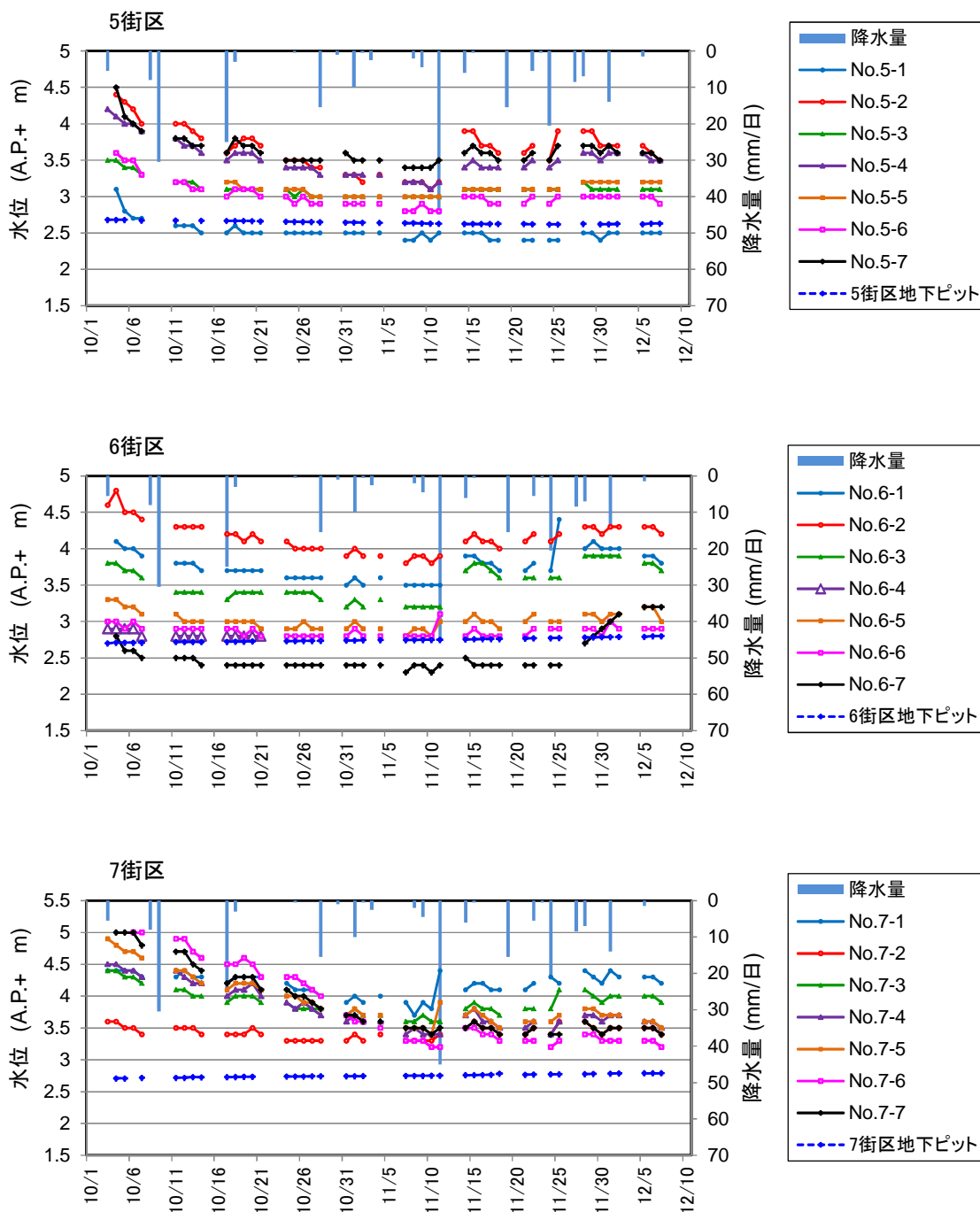
地下水水位および地下ピット内水位の変化
