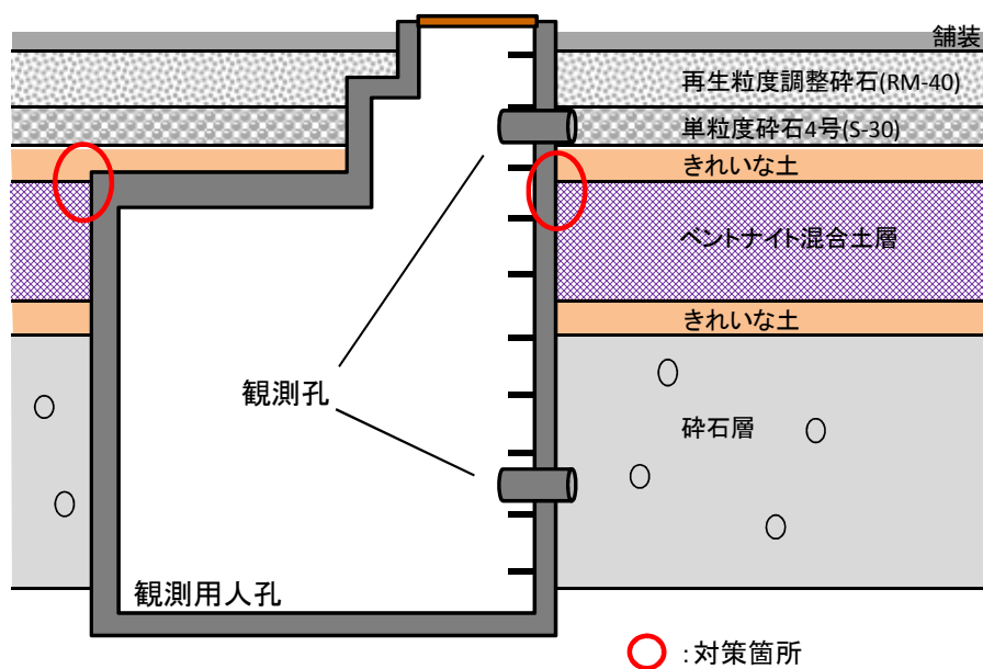
断面イメージ図
